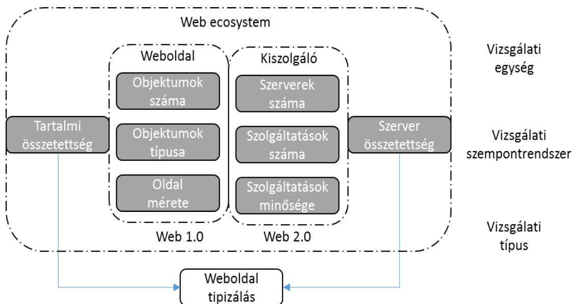
28. ábra Butkiewicz modelljének sémája (Forrás: Butkiewicz et al. 2011 alapján, saját szerkesztés)
