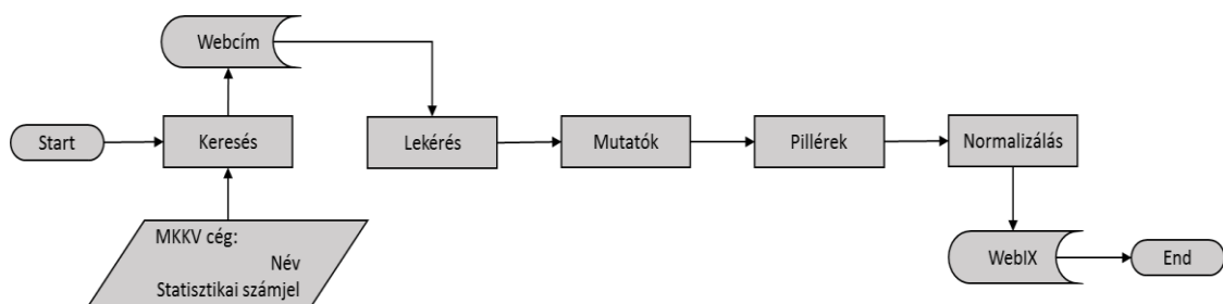
30. ábra WebIX számítási folyamata (Forrás: saját szerkesztés)
